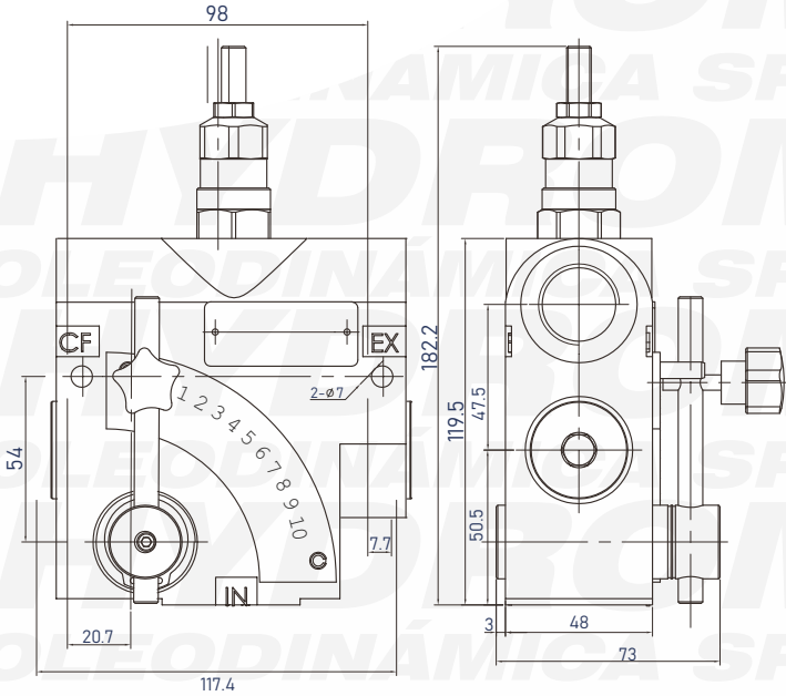
Válvula Reguladora de Caudal con Alivio Fijo /Flow regulator valve with relief valve
