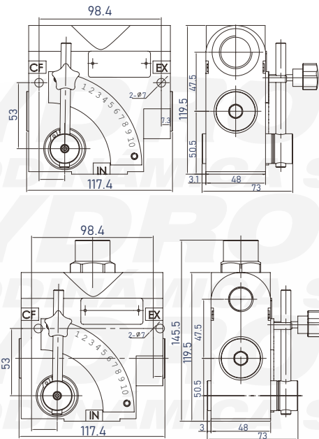
Válvula Reguladora de Caudal Standard /standard flow regulator valve
